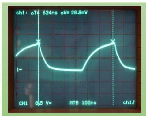
Figure 5 : oscillogramme du signal en sortie de l'oscillateur PO – Fréquence maxi.
