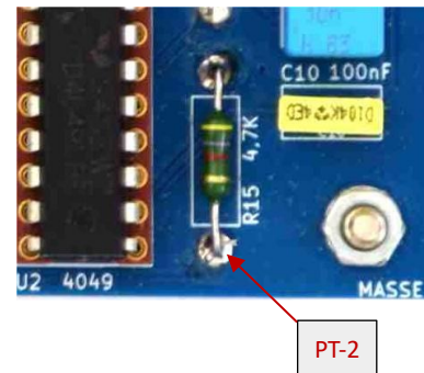
Figure 6 : repérage du point test PT-2.
