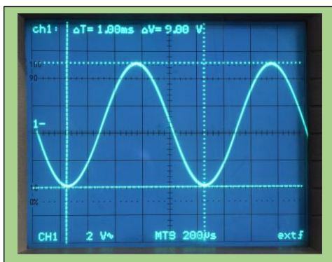
Figure 18 : oscillogramme du signal AF à la sortie du circuit TL071 (PT-7) et à la sortie du modulateur (PT-8).
