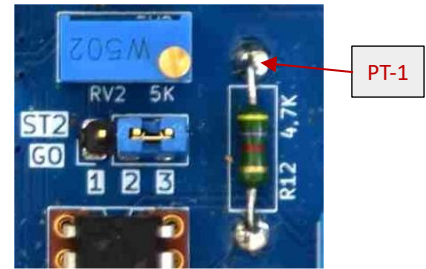
Figure 3 : repérage du point test PT-1.
