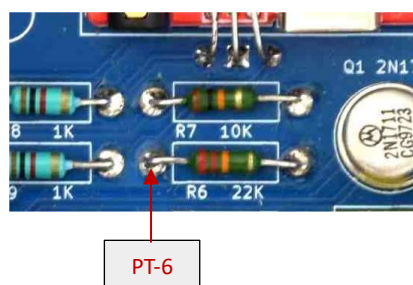
Figure 15 : repérage de PT-6.
