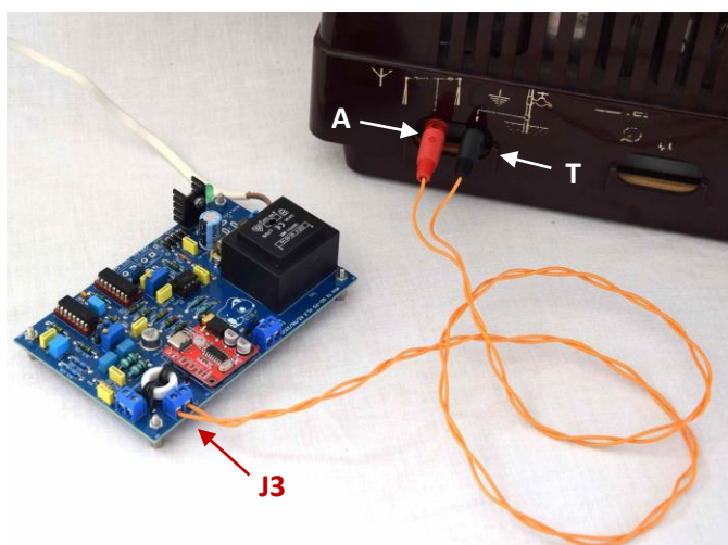
Figure III-07 : raccordement de la sortie RF symétrique, via le bornier J3, vers les bornes Antenne et Terre d'un poste récepteur AM.
