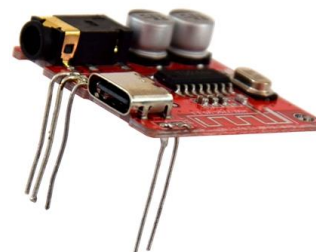
Figure II-08 : module Bluetooth, une fois préparé.
