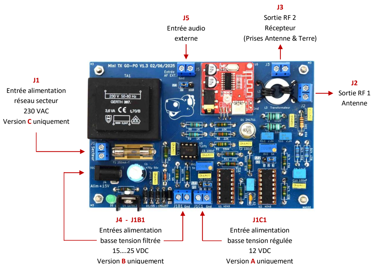
Figure III-03 : repérage des connecteurs (pour l'illustration, le module est câblé ici en toutes versions).
