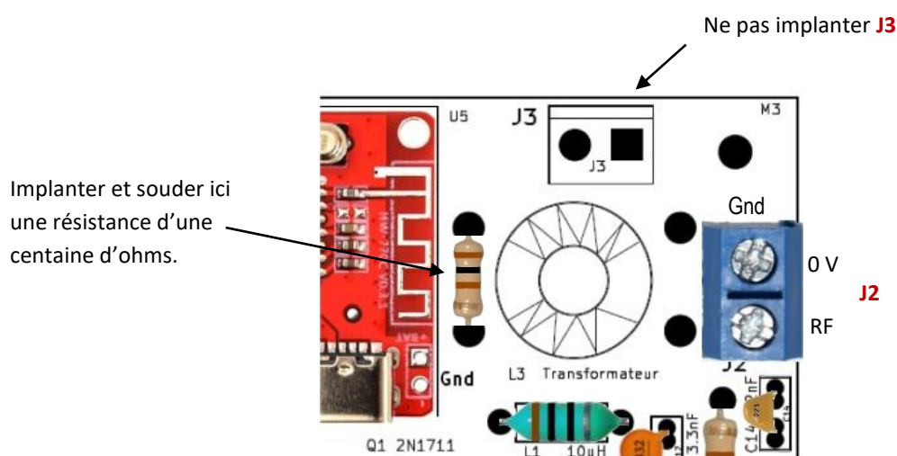
Figure V-02 : variante de câblage : seule la sortie RF asymétrique ( J2 ) est câblée.
