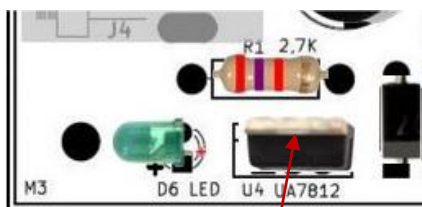
Circuit imprimé v1.3 et antérieur.
